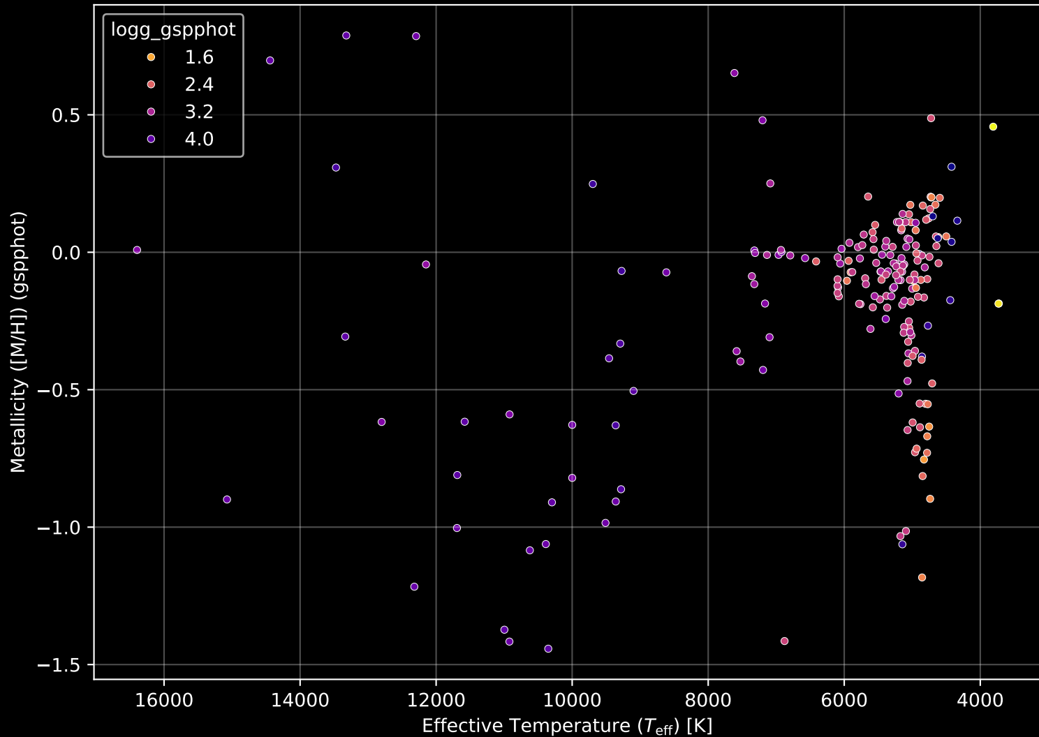
APOGEE DR17 Field: [225-04] Stellar Population Parameters (n= 206)
